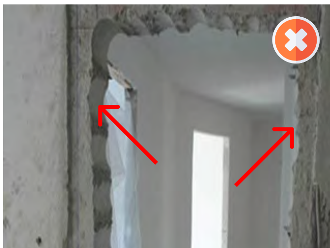
Проем не прямоугольной формы с наплывом раствора
